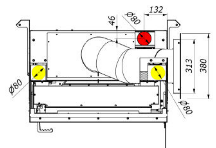
INSERT + RÉSERVE SUPPLÉMENTAIRE PELLET + TUBE DE CHARGEMENT ORIENTABLE CHARGEMENT PELLET AVEC TRAPPE + PIEDS
