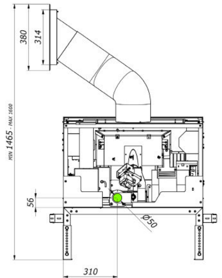
INSERT + TUBE DE CHARGEMENT
