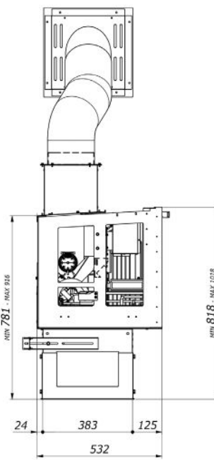
INSERT + RÉSERVE SUPPLÉMENTAIRE PELLET + TUBE DE CHARGEMENT ORIENTABLE CHARGEMENT PELLET AVEC TRAPPE + PIEDS
